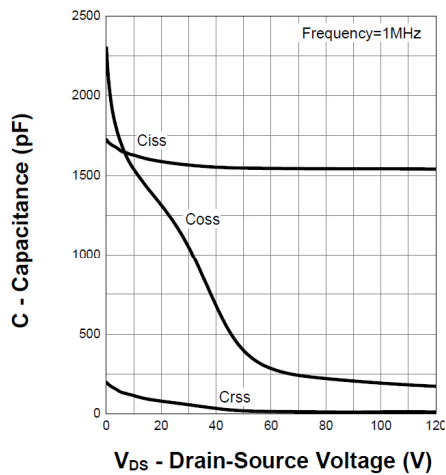
Fig 11. Capacitance
