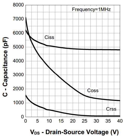
11. Capacitance
